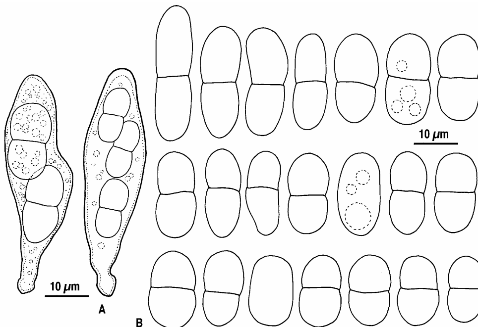
Fig. 5. Lichenochora paucispora (Holótipo).- A, ascos. B, ascósporas.
